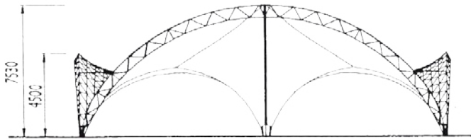
PROSPETTO FRONTALE
