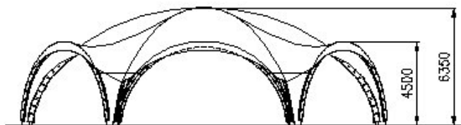
VISTA FRONTALE
